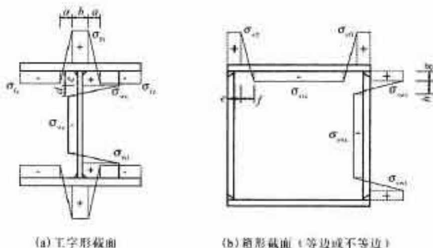
图 4 焊接构件的残余应力分布模式(清华大学)
