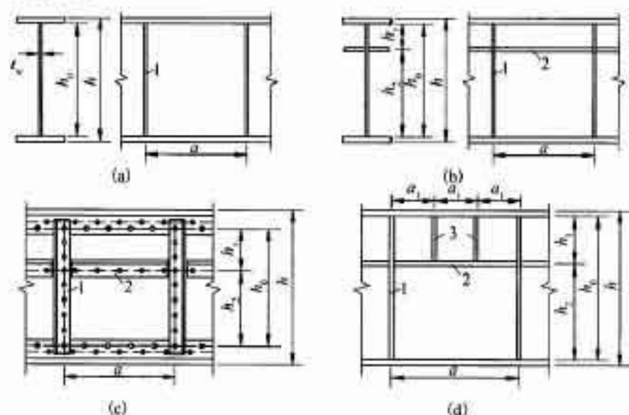
图 5.3.10 加劲肋布置
