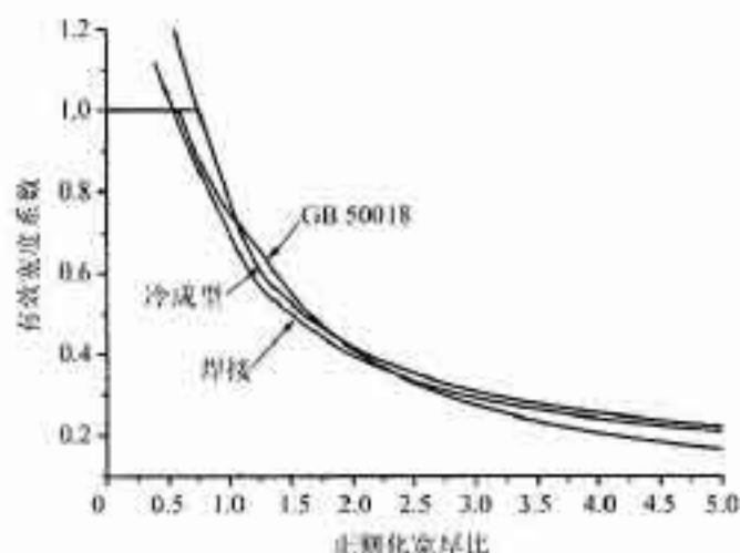
图 8 本规程中有效宽度系数曲线与 GB 50018 中曲线对比
