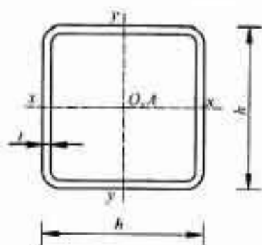
图 B.1.1 方钢管截面特性示意图
