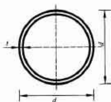
图 B.1.2 薄壁圆钢管截面特性示意图
