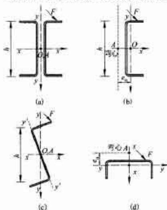
图 5.3.8 荷载偏离弯心且与主轴倾斜的受弯构件截面示意图
