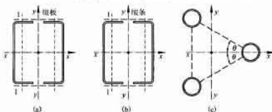
图 5.2.6 格构式构件截面示意图
