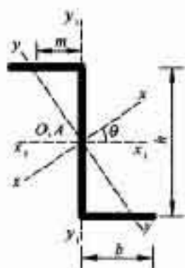
图 B. 2. 7 Z 型钢截面特性示意图
