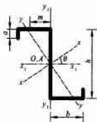
图 B. 2. 8 卷边 Z 型钢截面特性示意图
