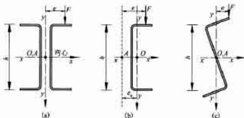
图 5.3.7 荷载偏离弯心但与主轴平行的受弯构件截面示意图
