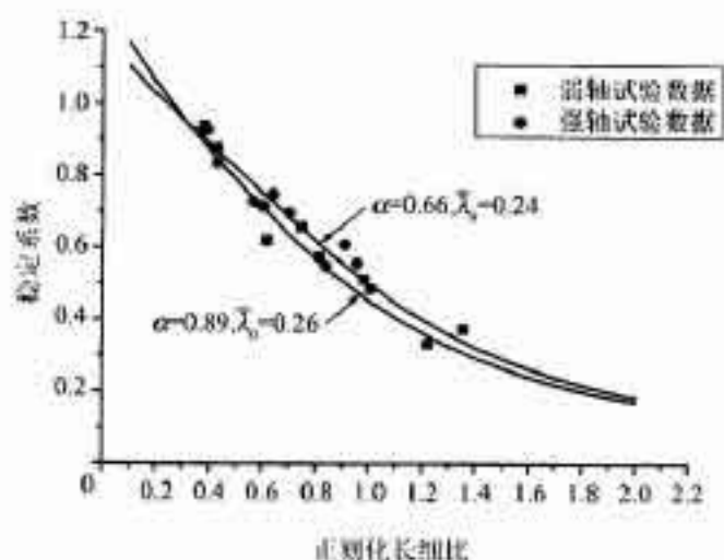
图 3 奥氏体型焊接 H 形截面柱子曲线和试验数据对比
