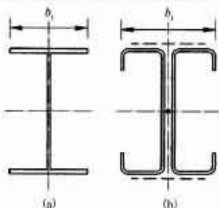
图 5.3.3 典型截面的翼缘宽度 b_1
