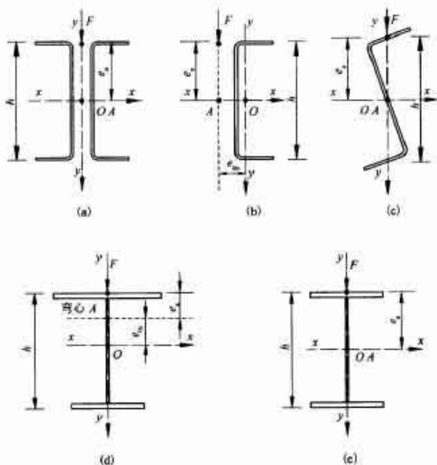
图 A. 0.1 典型单轴和双轴对称截面
