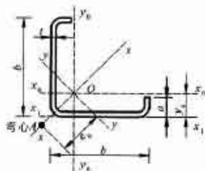
图 B.1.4 卷边等边角钢截面特性示意图
