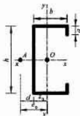
图 B. 2. 6 向内卷边槽钢截面特性示意图
