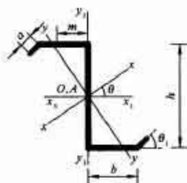
图 B. 2. 9 斜卷边 Z 型钢截面特性示意图
