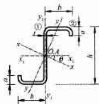
图 B.1.7 卷边 Z 型钢截面特性示意图
