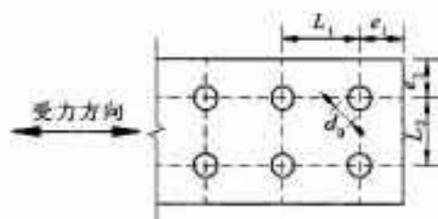
图 6.2.6 不锈钢抽芯铆钉连接的边距、端距和间距示意图
