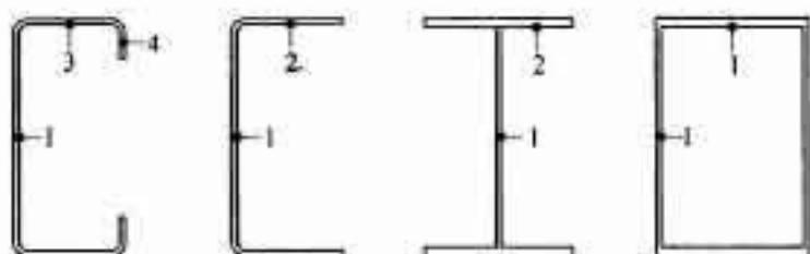
图1 构件中受压板件的分类
