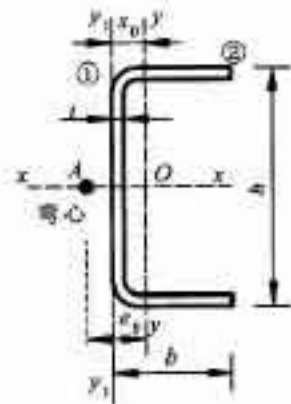
图 B.1.5 槽型截面特性示意图
