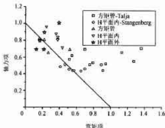
图7 压弯构件试验数据与按本规程计算结果对比
