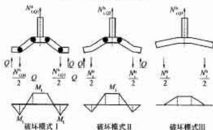
图10 T形连接的破坏模型
