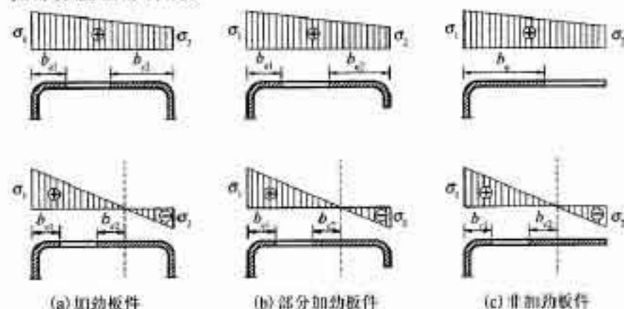
图 5.6.5 受压板件的有效截面图
