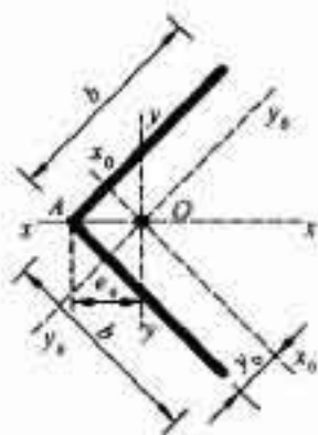
图 B. 2. 2 等边角钢截面特性示意图
