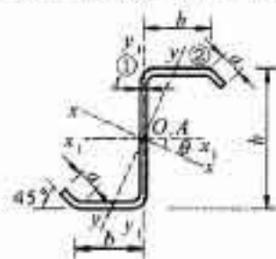
图 B.1.8 斜卷边 Z 型钢截面特性示意图
