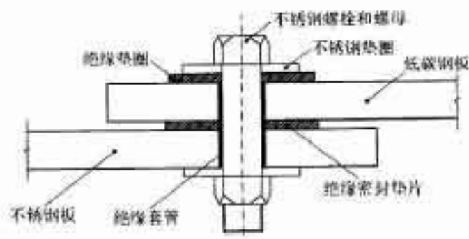
图 11 低碳钢板和不锈钢板螺栓连接示意图
