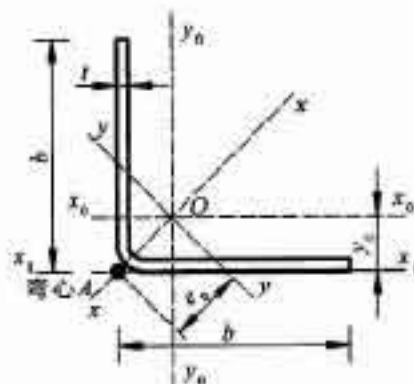
B.1.3 等边角钢截面特性示意图
