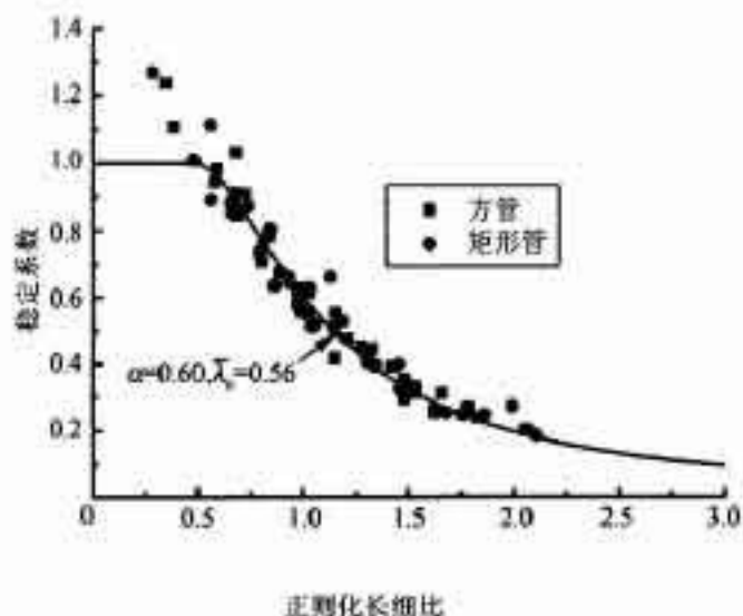
图 2 冷成型方矩管构件试验数据与柱子曲线对比
