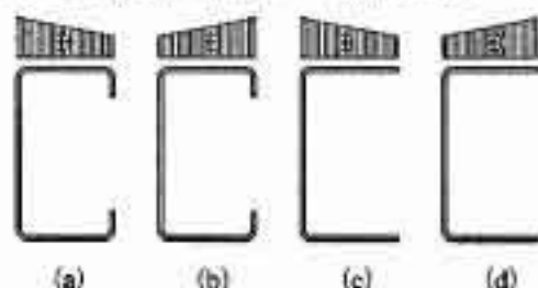
图 5.6.3 部分加劲板件和非加劲板件的应力分布示意图
