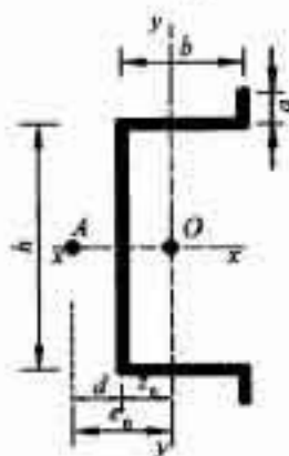
图 B. 2. 5 向外卷边槽钢截面特性示意图
