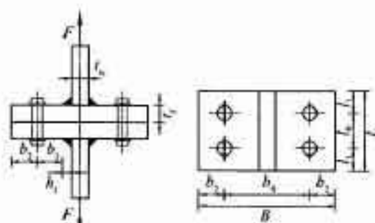
图9 T形构件受拉螺栓连接
