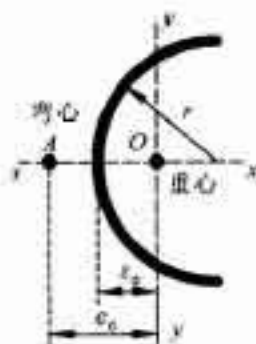
图 B.2.1 半圆钢管截面特性示意图
