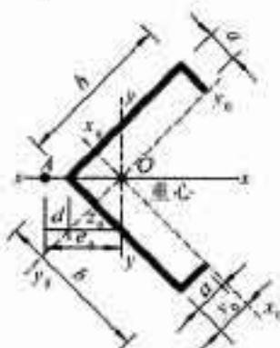
图 B. 2. 3 卷边等边角钢截面特性示意图
