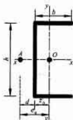
图 B. 2. 4 槽钢截面特性示意图
