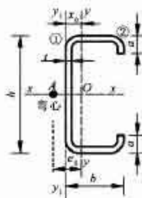
图 B.1.6 卷边槽型截面特性示意图
