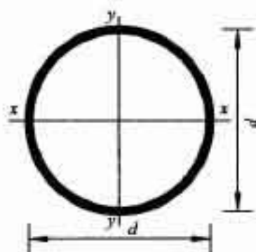
图 B. 2. 10 圆钢管截面特性示意图
