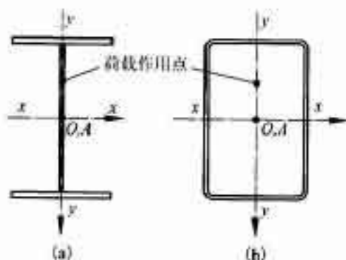
图 5.5.2 双轴对称截面示意图
