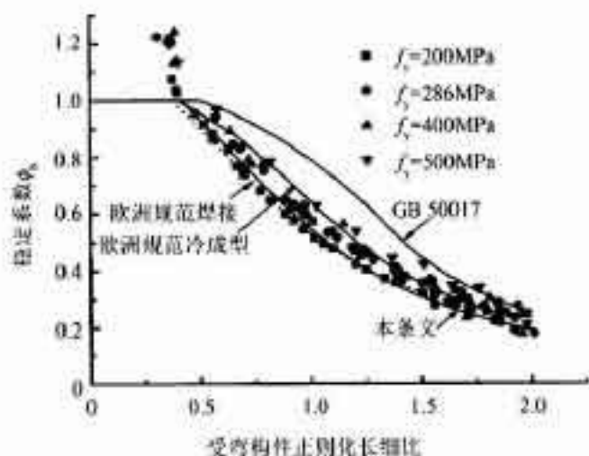
图6 梁整体稳定系数与有限元分析结果对比
