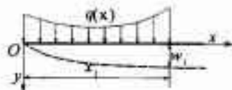
图 5.7.1 受弯构件变形的计算简图
