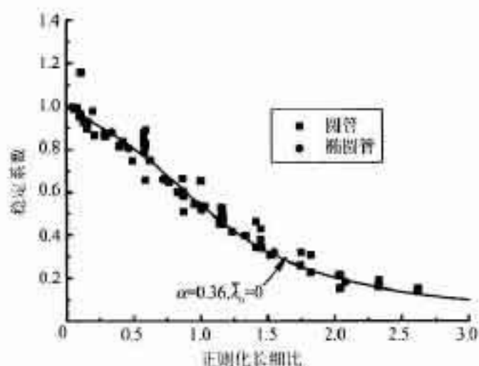
图 3 冷成型圆管构件试验数据与柱子曲线对比
